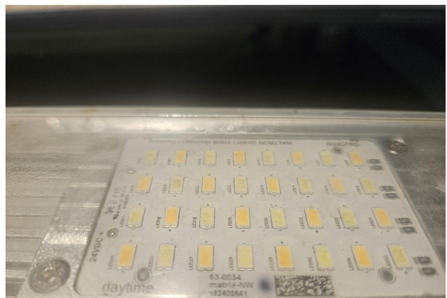
LED-Modul Daytime matrix-NW (insgesamt 18 Module)
